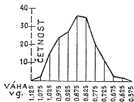
Obr. č. 2. Diagram vahových četností 6. typu řezenských feniků z nálezů ve Stříbře.
