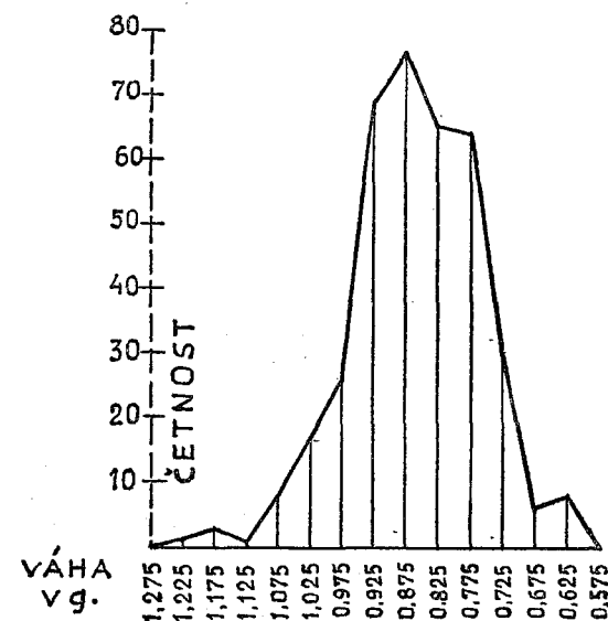
Obr. č. 1. Diagram vahových četností 5. typu řezenských feniků z nálezu ve Stříbře.
