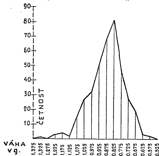
Obr. č. 4. Diagram vahových četností 8. typu řezenských feniků z nálezů ve Stříbře.
