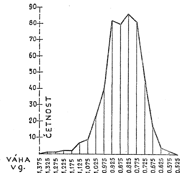
Obr. č. 3. Diagram vahových četností 7. typu řezenských feniků z nálezů ve Stříbře.
