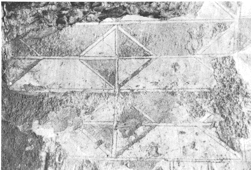
Obr. 20: Detail zbytků sgrafitové výzdoby uvnitř severního pilíře arkády pozdně gotické budovy.
