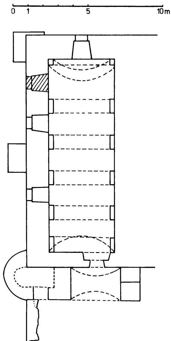
Obr. 13: Polánka, současný stav severní části pozdně gotické budovy s Petráňkou a opěrnými pilíři (měřeno 23. 7. 1994).
