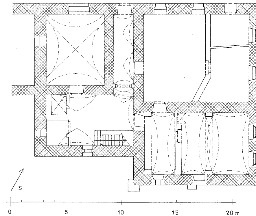
Obr. 3: Dub (Tábor), plán přízemí budovy tvrze. Křížky je vyznačeno předpokládané středověké zdivo, mladší konstrukce nejsou rozlišeny. Stav 8. července 2000, zaměření Helena Klímová a autor, kresba autor.
