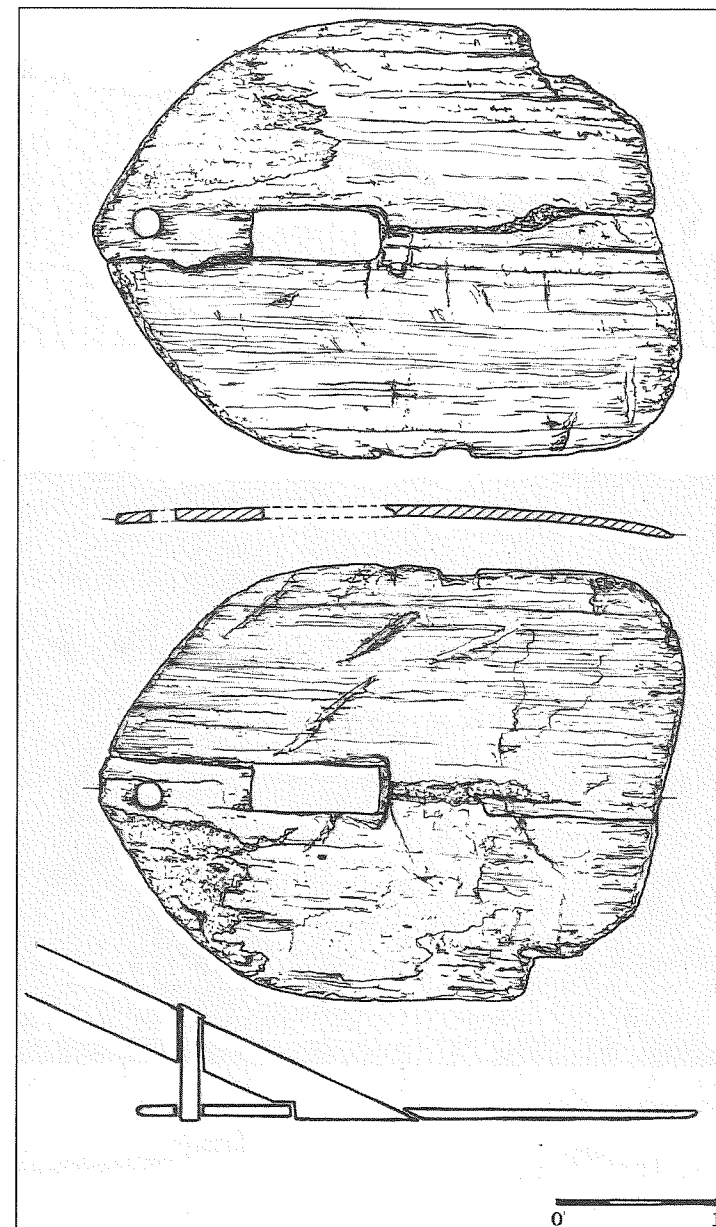
Obr. 1. Horní a spodní pohled a řez dřevěným artefaktem i.č. SA 12 710, Husitské muzeum v Táboře. Rekonstrukční schéma připojení násady k pracovní desce tábor-ské středověké lopaty.
