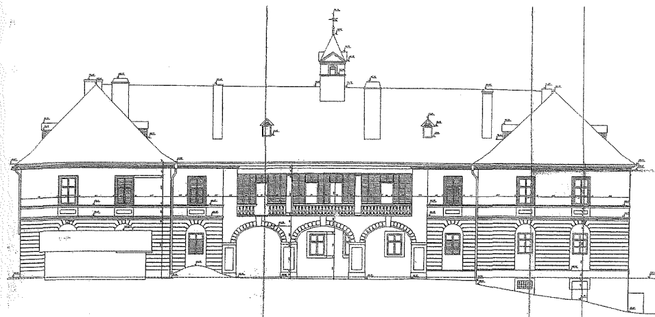
Obr. 9. Přehořov (okr. Tábor), severní zámecké průčelí. Zaměření provedla Inženýrská Geodézie, n. p. Praha, závod České Budějovice v roce 1968. Originál uložen v Národním památkovém ústavu, územním odborném pracovišti v Českých Budějovicích.
