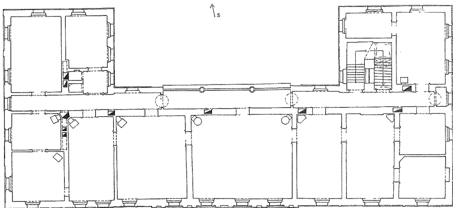
Obr. 7. Přehořov (okr. Tábor), plán patra zámku. Zaměření provedla Inženýrská Geodézie, n. p. Praha, závod České Budějovice v roce 1968. Originál uložen v Národním památkovém ústavu, územním odborném pracovišti v Českých Budějovicích, kresba autor.
