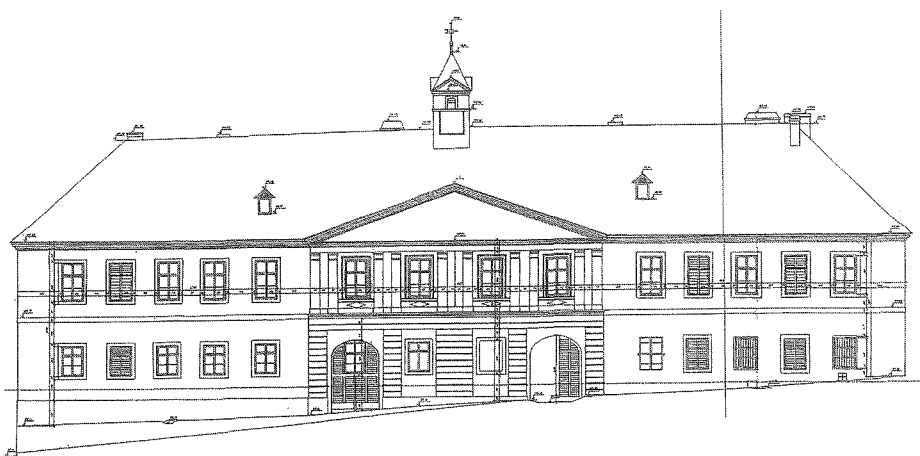
Obr. 8. Přehořov (okr. Tábor), jižní zámecké průčelí. Zaměření provedla Inženýrská Geodézie, n. p. Praha, závod České Budějovice v roce 1968. Originál uložen v Národním památkovém ústavu, územním odborném pracovišti v Českých Budějovicích.
