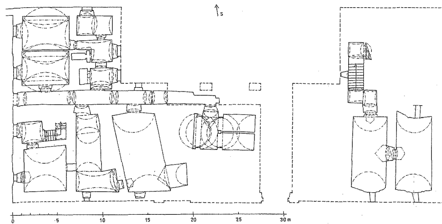
Obr. 5. Přešovice (okr. Tábor), plán sklepů zámku. Zaměření provedla Inženýrská Geodézie, n. p. Praha, závod České Budějovice v roce 1968. Originál uložen v Národním památkovém ústavu, územním odborném pracovišti v Českých Budějovicích, kresba autor.
