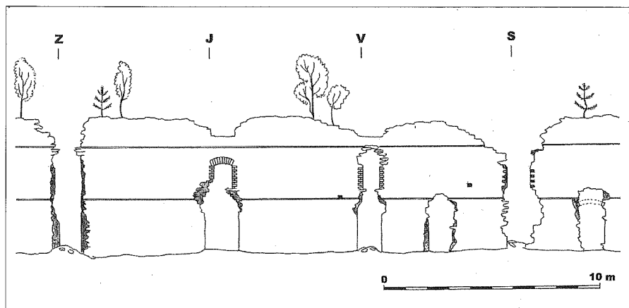
8. Rozvinutý pohled na vnější plášť zříceniny větrného mlýna. Zaměření a kresba autor, 2010.
