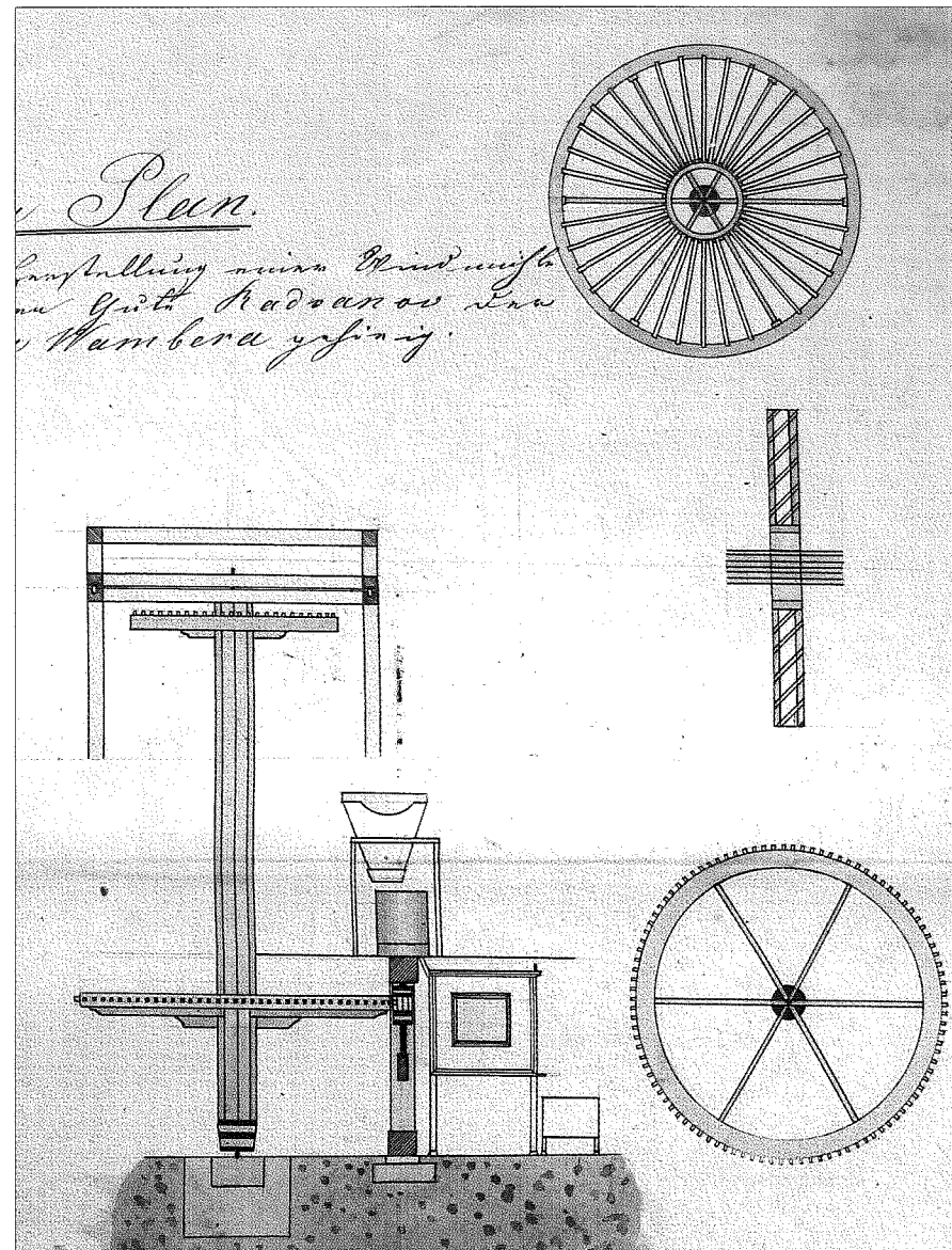
6. Detail stavebního výkresu – technické provedení svislé hřídele s mechanismem převodu otáčivého pohybu na cévové kolečko, pohánějící mlecí zařízení.
