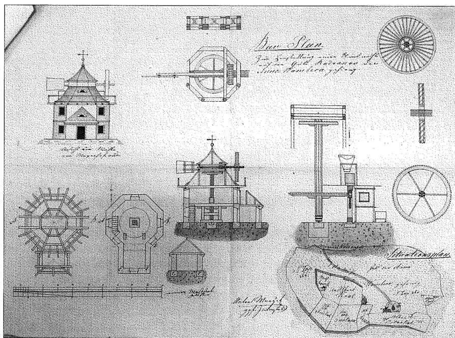
1. Radvanov – stavební plán větrného mlýna z roku 1855. Státní okresní archiv Tábor.
