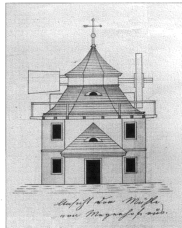
3. Detail stavebního výkresu – celkový pohled na budovu mlýna od jihu.
