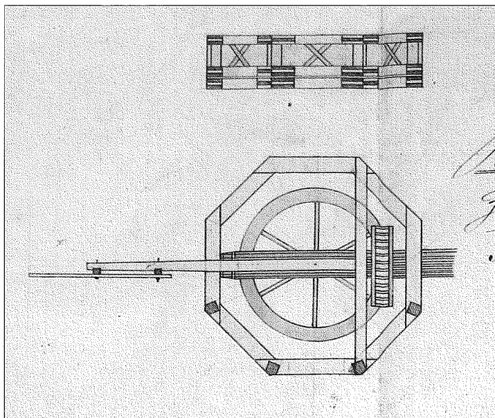
5. Detail stavebního výkresu – otočný střešní nástavec s mechanismem převodu otáčení z hřídele větrného kola na palečné kolo. Nahoře bokorys se schématem tesařského provedení.
