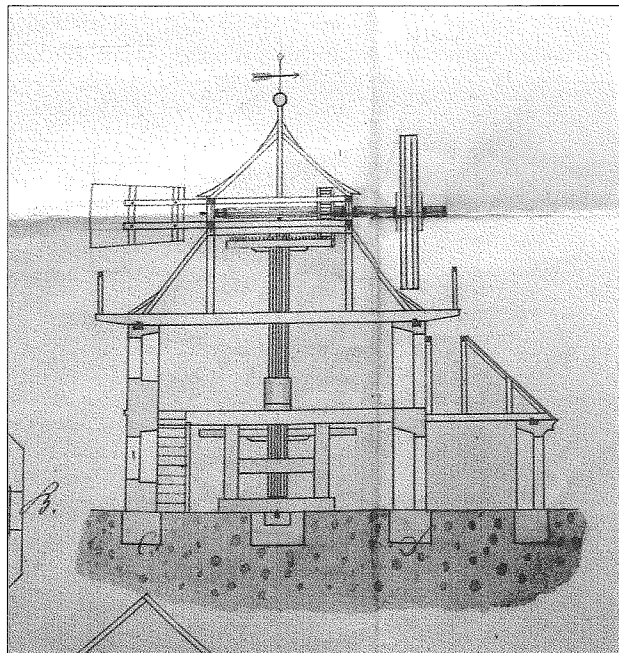
4. Detail stavebního výkresu – svislý řez budovou mlýna při pohledu od západu.
