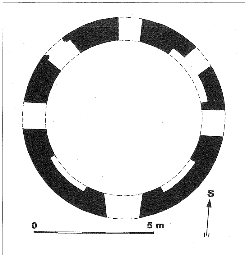
7. Půdorys zříceniny větrného mlýna nad Radvanovem v úrovni přízemí. Zaměření a kresba autor, 2010.
