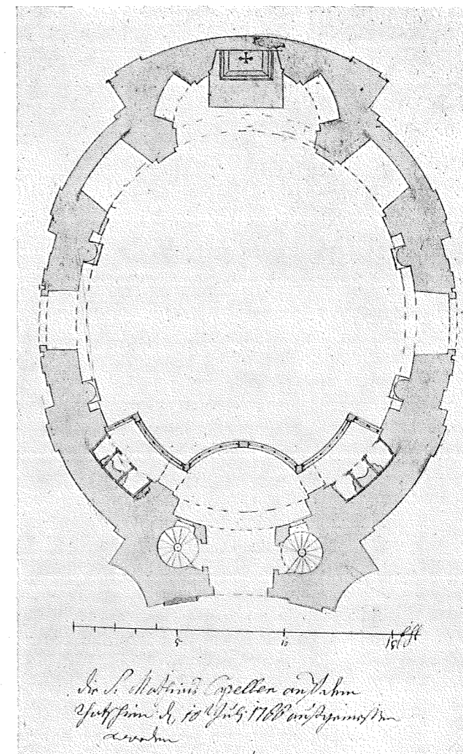
PŮDORYS KAPLE SV. MATOUŠE NA HRADČANECH.
