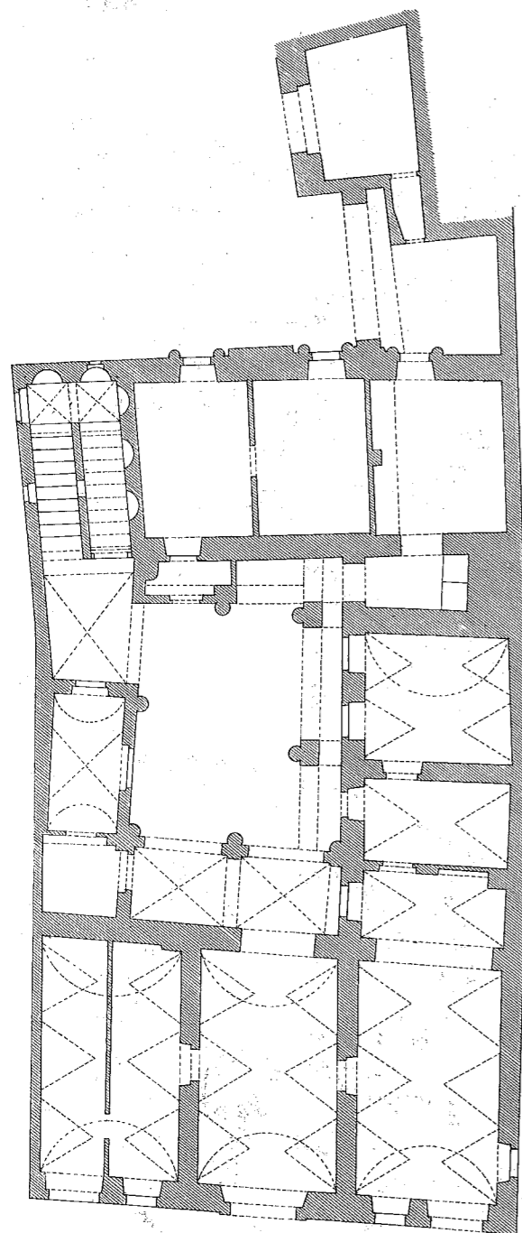
PŮDORYS PRŮZEMÍ Č. P. 73-V.
